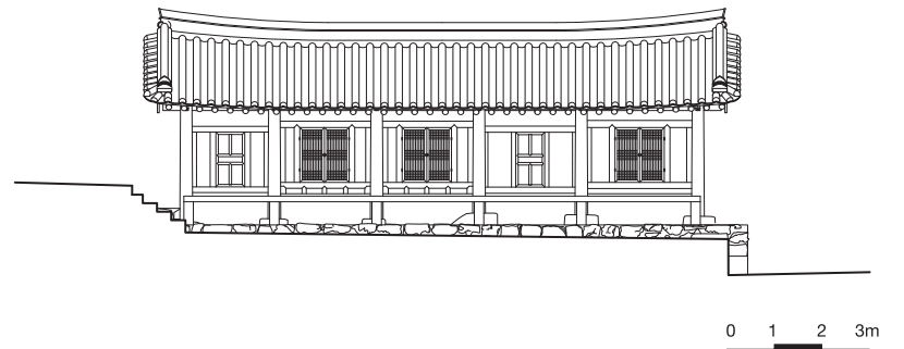
입면도
