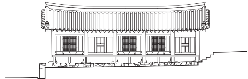
입면도
